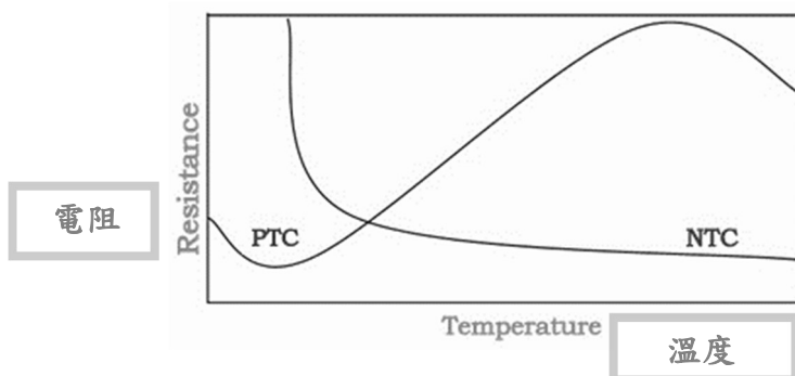
<熱敏電阻—溫度及電阻關係示意圖>
