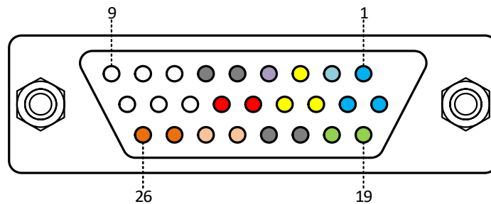
驅動器端 DB26 母連接頭
