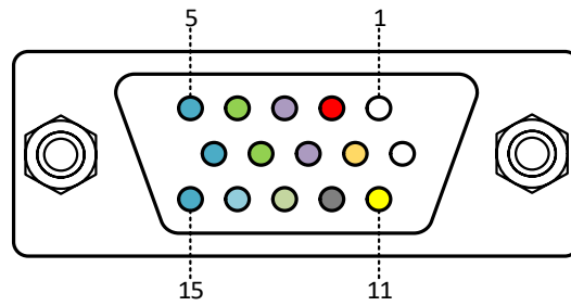
驅動器之 DB15 母連接器
