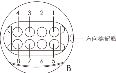
彈簧探針
