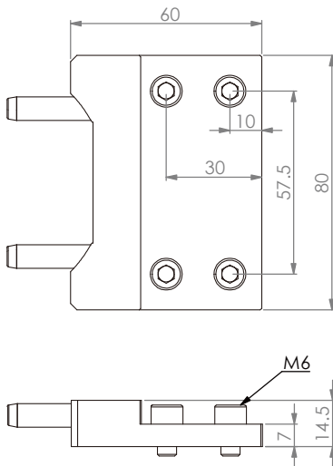
換刀固定座
