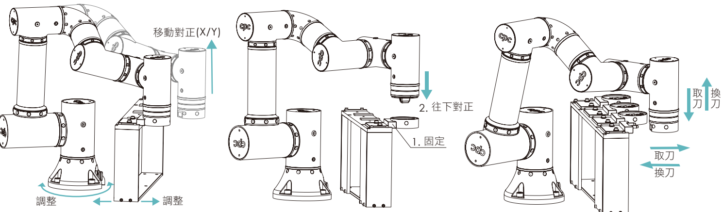
設定換刀機構與機械手臂座標之對正
