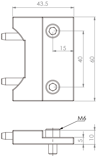
換刀固定座
