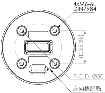
手臂末端連接板
