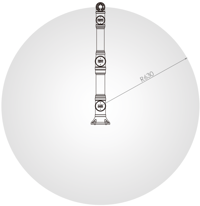
運動區域
