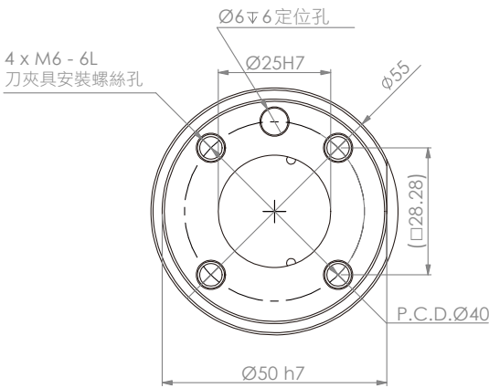
工具側連接板尺寸
