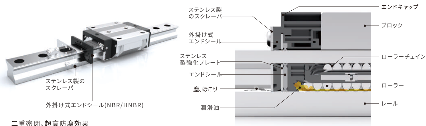
二重密閉、超高防塵効果
