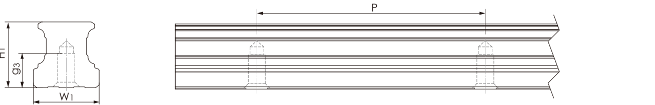
ARU Series 下取付け式レール
