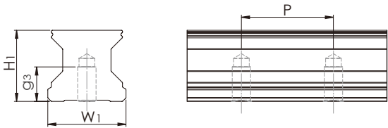
ARRU Series 下取付け式レール
