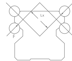
Xタイプ アレンジメント
